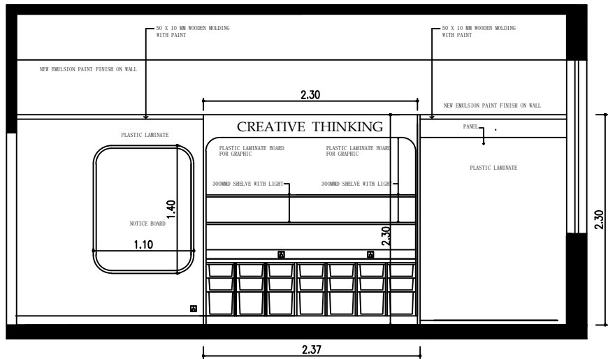
ELEVATION BB
