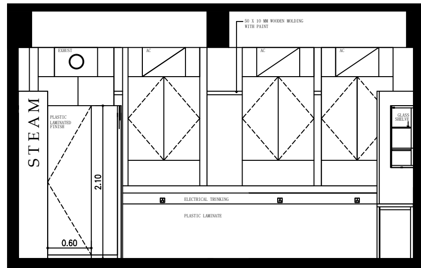
ELEVATION DD
